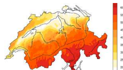
Durée moyenne d'ensoleillement en janvier en Suisse.
